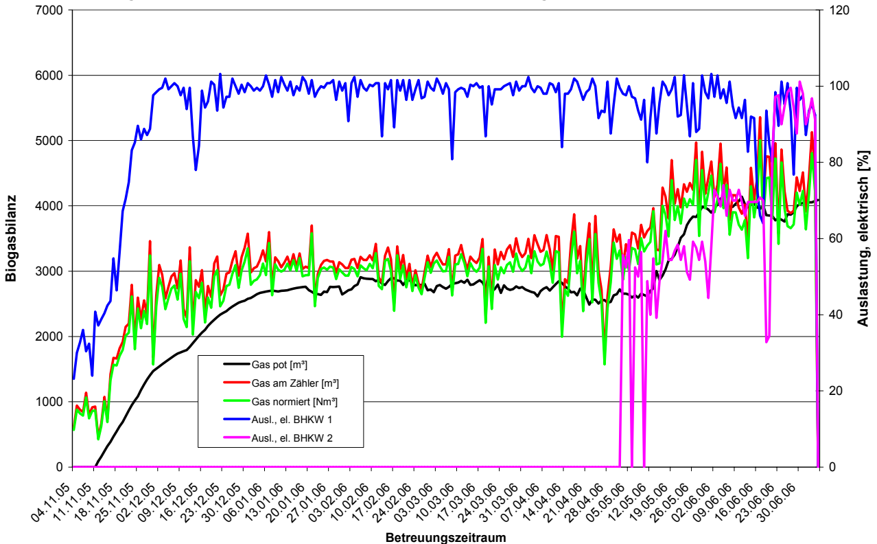
Abb.: Auslastung der Blockheizkraftwerke seit Inbetriebnahme der Anlage.
